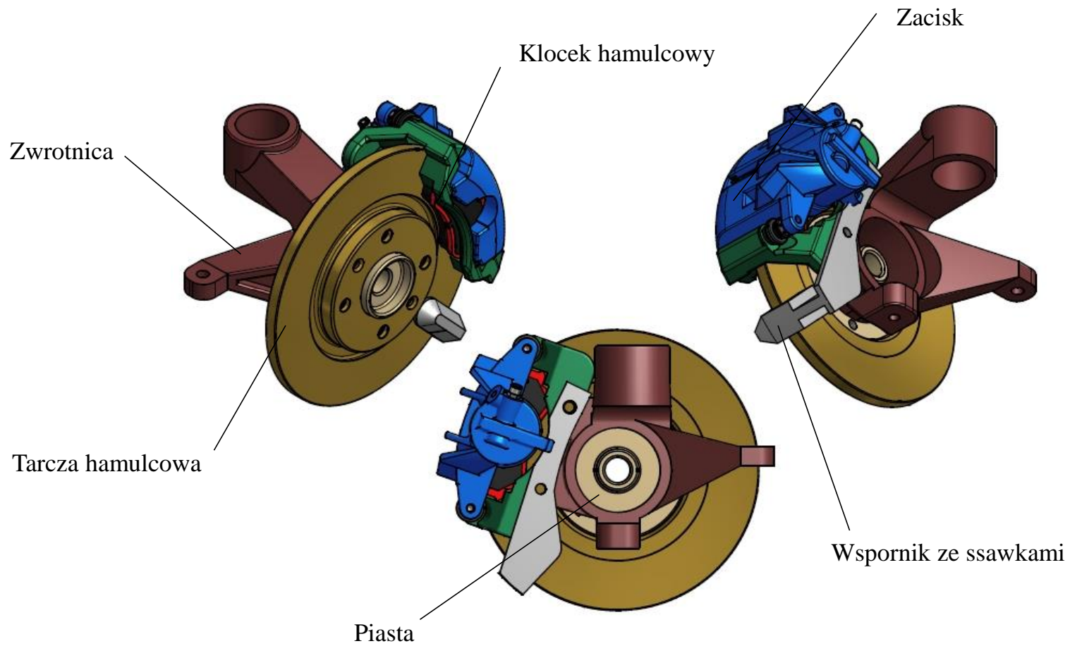
Schemat zamocowania urządzenia do zmniejszania emisji pyłu hamulcowego do zwrotnicy koła
